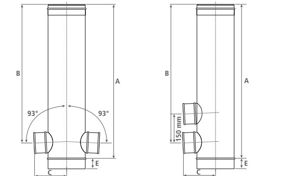
I Té 93° double débouchure à 180° J Té 93° double débouchure parallèle
