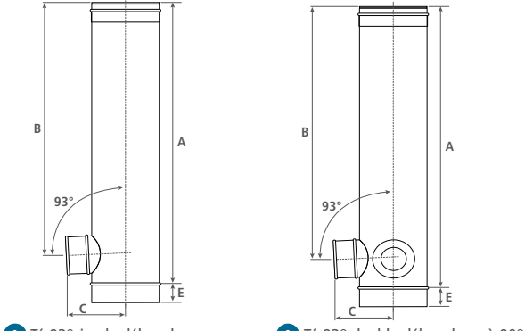
I Té 93° simple débouchure J Té 93° double débouchure à 90°
