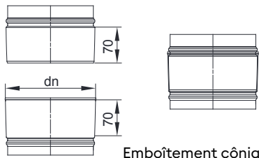
Emboîtement cône
